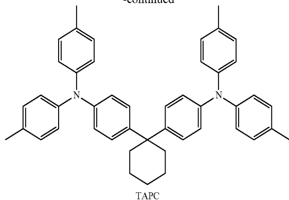
TAPC
