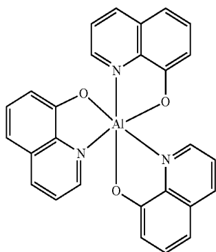
Alq 3
