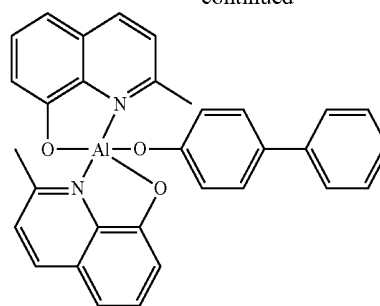
Balq
